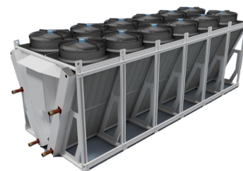
V-образное исполнение
